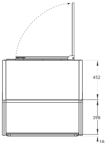
Vista superior
