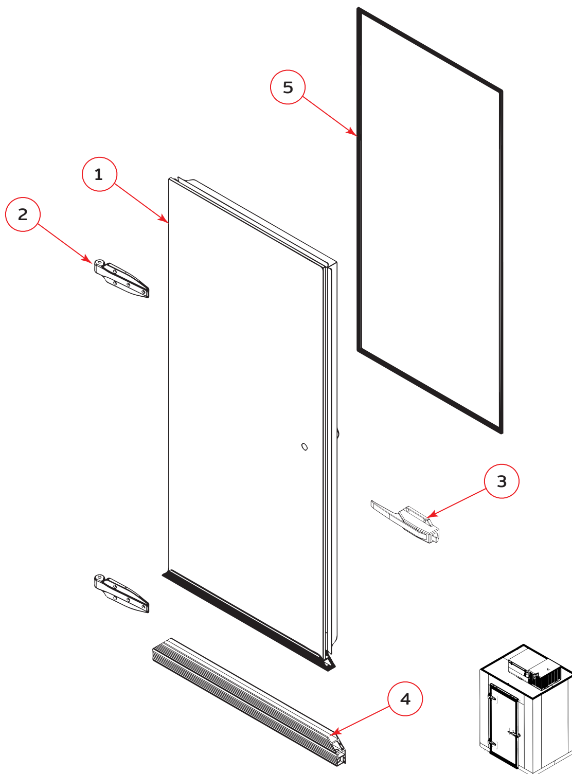
ENSAMBLE DE PUERTA
